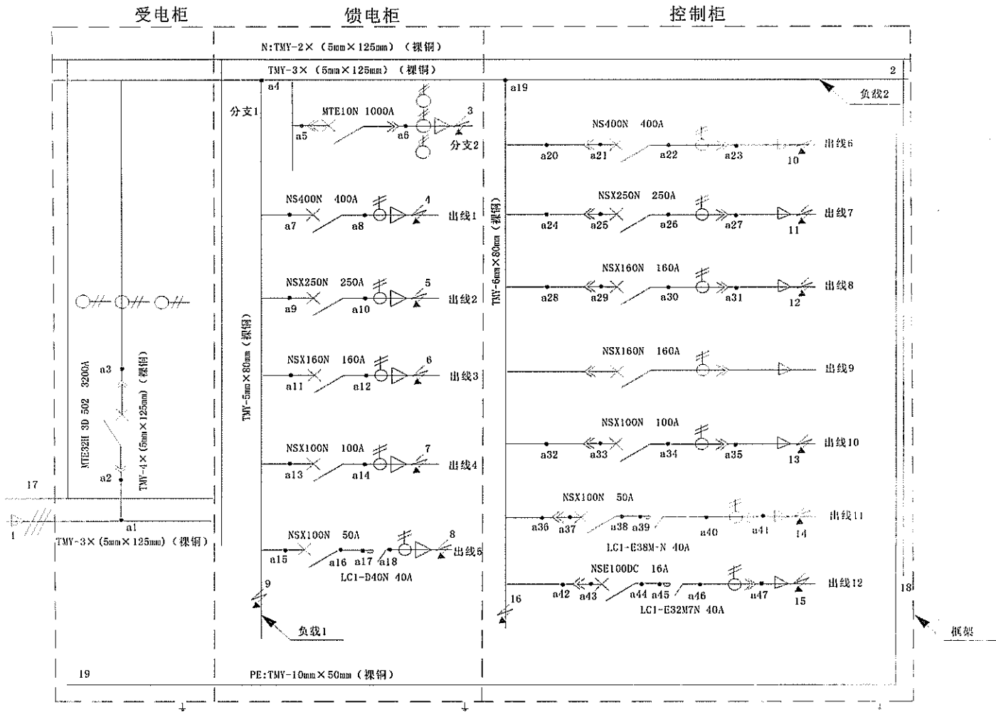
温升、短路点示意图 F1
