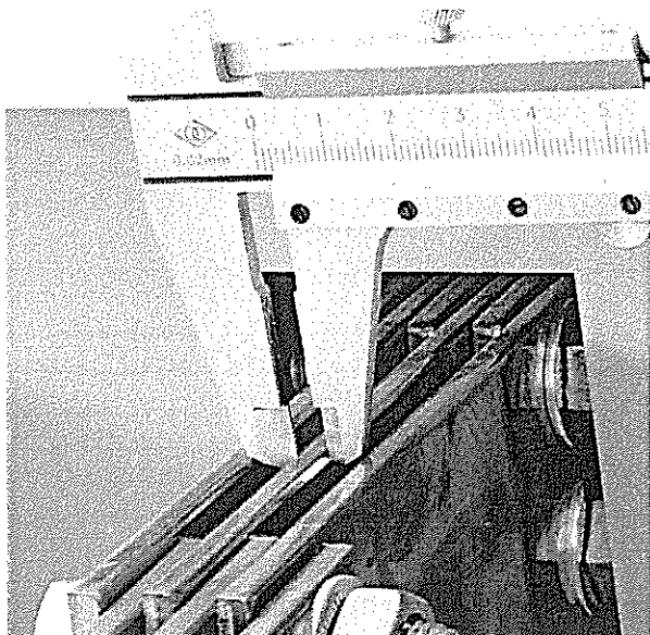
水平母线厚度照片
