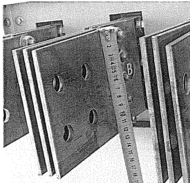
水平母线宽度照片
