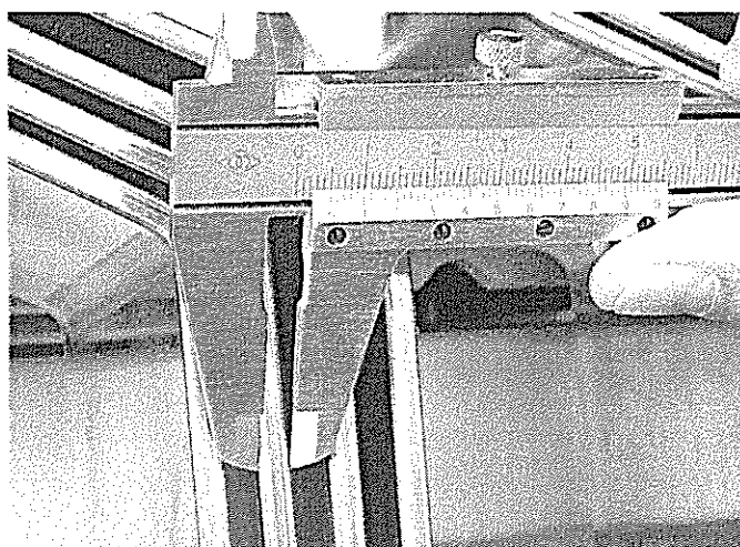
主断路器进出线厚度照片
