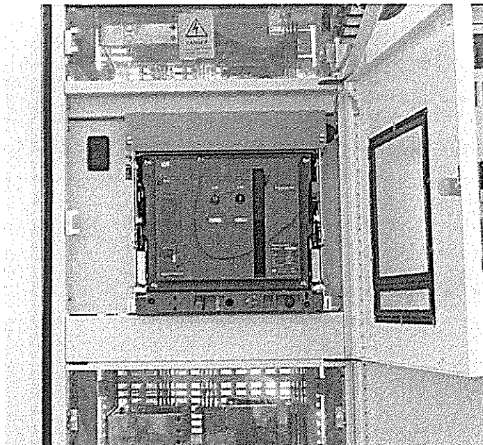
主断路器照片
