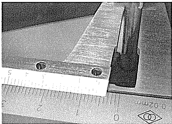
控制柜配电母线厚度照片
